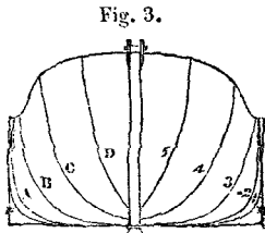
Body Plan.
