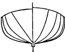
BODY PLAN.
