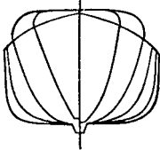
BODY PLAN.
