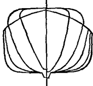
BODY PLAN.
