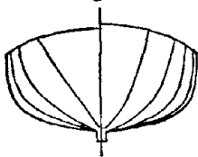
BODY PLAN.
