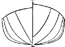
BODY PLAN.
