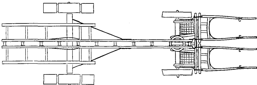
PLAN.
