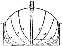
Body Plan.
