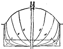
Body Plan.
