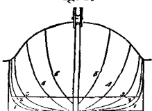
Body Plan.
