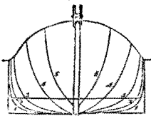
Body Plan.
