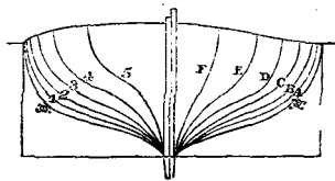
Body Plan.
