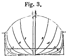
Body Plan.
